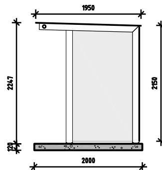
tVÄRSNITT
